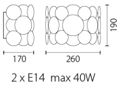
2 x E14 max 40W
