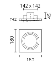
1 x AR111 max 50W
