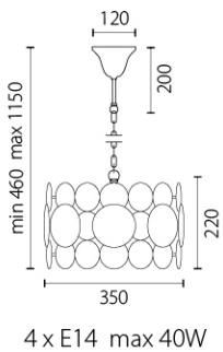
4 x E14 max 40W
