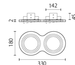
2 x AR111 max 50W
