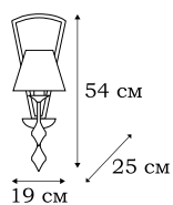
■ L15021.37 1 x E14 (60W)
