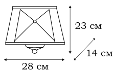
■ L57722.32 2 x E14 (60W)
