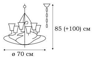
■ L55606.17 6 x E27 (60W)
