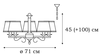
■ L12105.88 5 x E14 (60W)
