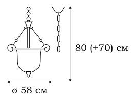
■ L50303.46 3 x E14 (60W)
