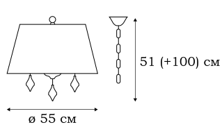
■ L15015.37 5 x E14 (60W)
