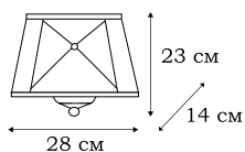
■ L57722.88 2 x E14 (60W)
