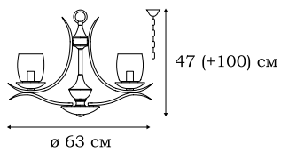
■ L22003.26 3 x E14 (60W)
