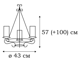
■ L18203.10 3 x E14 (60W)
