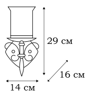
■ L14521.27 1 x E27 (60W)
