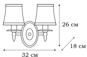
■ L10522.54 2 x E14 (40W)
