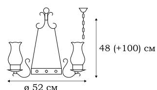
■ L11903.88 3 x E14 (60W)
