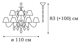
■ L15012.37 12 x E14 (60W)
