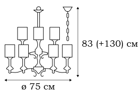
■ L50009.05 9 x E27 (60W)
