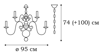
■ L19212.86 12 x E14 (60W)
