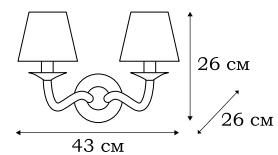
■ L14322.21 2 x E14 (60W)
