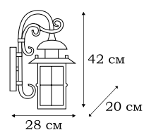
■ L70781.07 1 x E27 (100W), IP - 23
