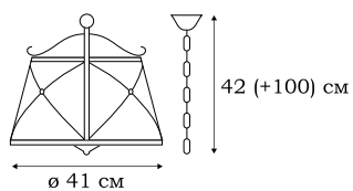
■ L57703.08 3 x E14 (60W)
