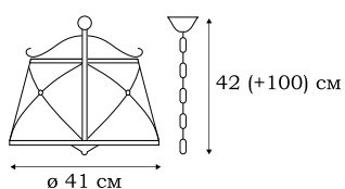
■ L57703.32 3 x E14 (60W)
