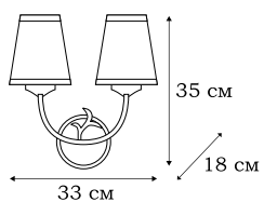
■ L17822.03 2 x E14 (60W)
