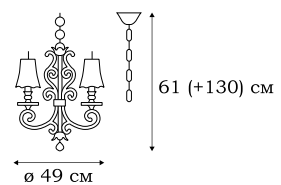
■ L54904.24 4 x E14 (60W)
