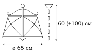
■ L57705.32 5 x E14 (60W)
