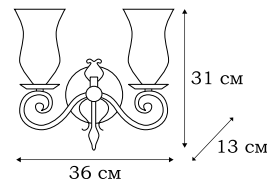
■ L12322.36 2 x E14 (60W)
