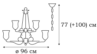
■ L17712.19 12 x E27 (60W)
