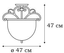
■ L17753.19 3 x E14 (60W)
