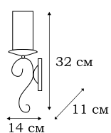
■ L18221.10 1 x E14 (60W)
