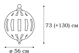
■ L50406.00 6 x E14 (60W)
