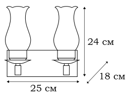
■ L11922.88 2 x E14 (60W)
